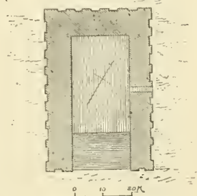
143. — Plan du temple de Moughéir, d'après Loftus.
